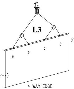
L3 4 WAY EDGE OR 4 WAY FACE (L3-F)
